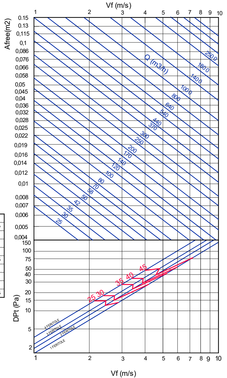
VELOCITA LIBERA, PERDITI DI CARICO, POTENZA SONORA
