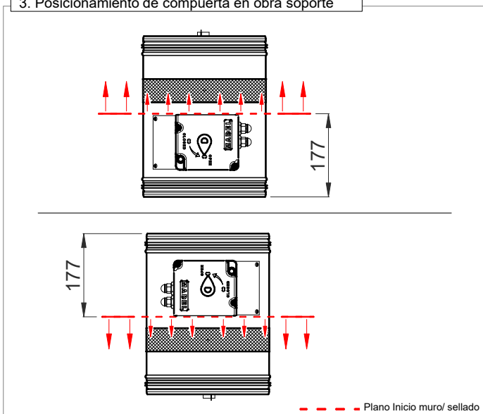
3. Posicionamiento de compuerta en obra soporte
