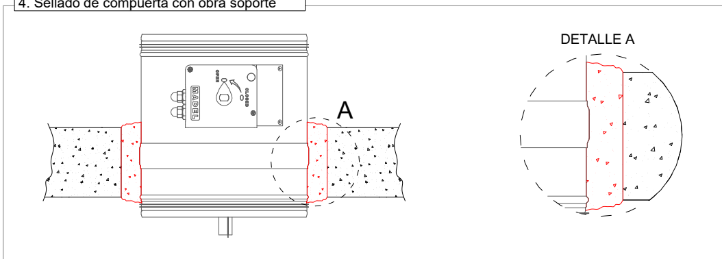
4. Sellado de compuerta con obra soporte
